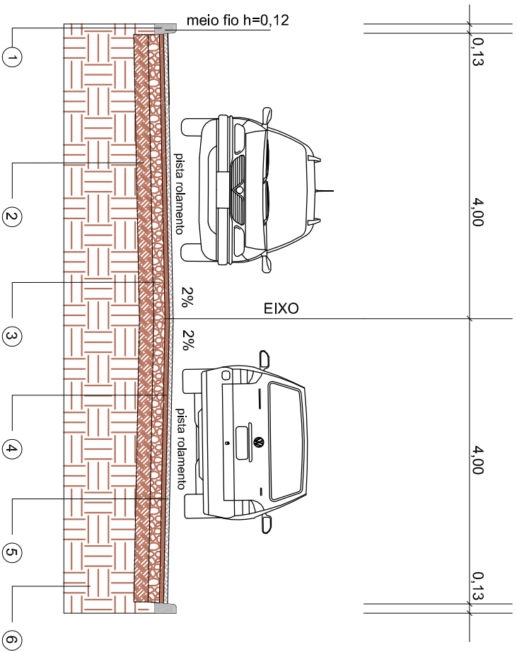
SEÇÃO-TIPO - PAVIMENTAÇÃO PVS
