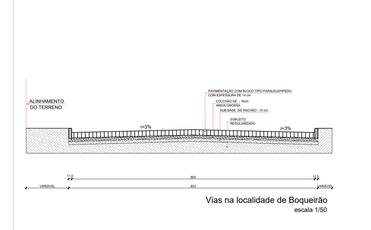
SEÇÃO DE PAVIMENTAÇÃO ESC. 1/75
