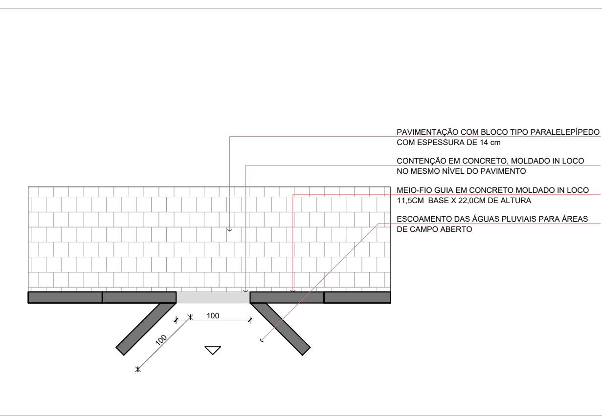
DETALHE SAÍDA PLUVIAL ESC. 1/50
